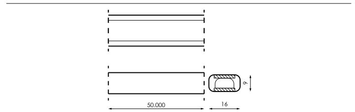
ESQUEMA DE DOBLADO
