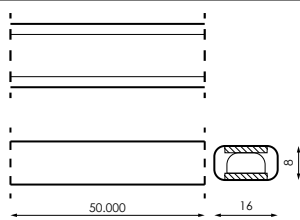
ESQUEMA DE DOBLADO
